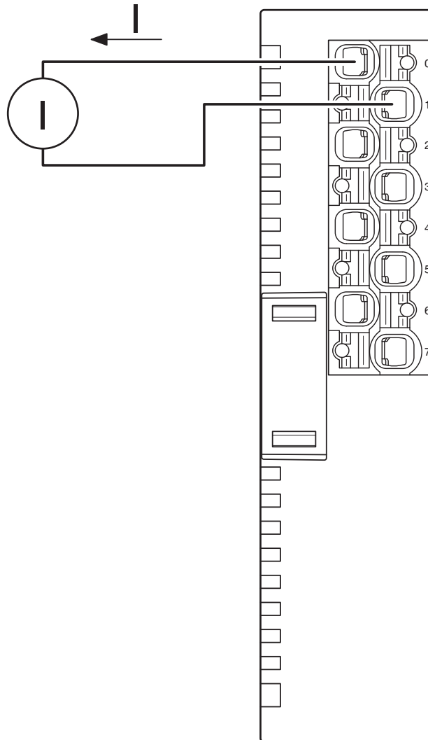
Disegno collegamento
