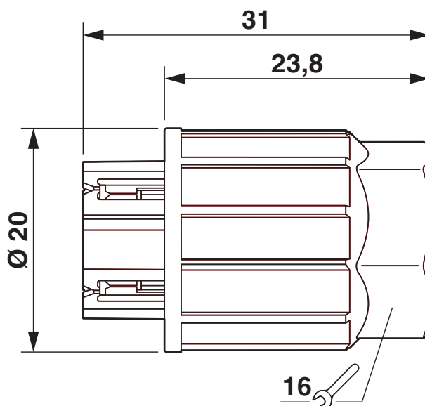
Disegno quotato
