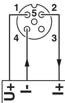
Disegno collegamento
