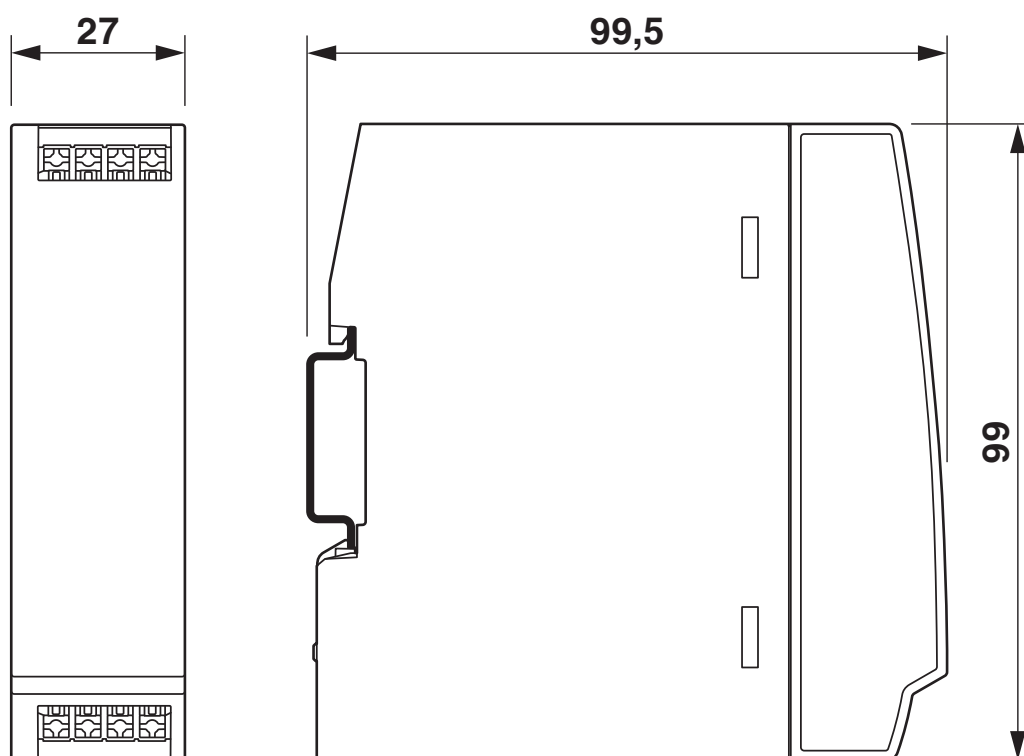
Disegno quotato
