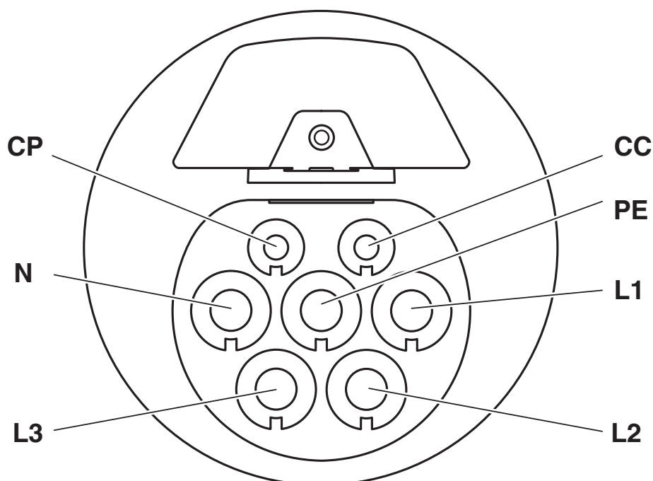
Disegno collegamento
