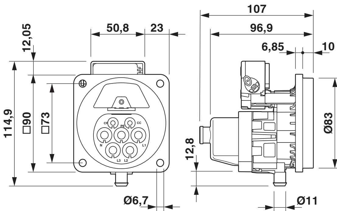
Disegno quotato
