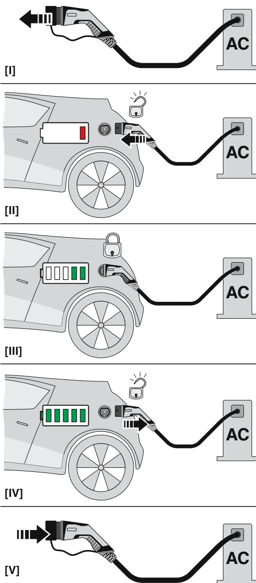
Disegno funzionamento
