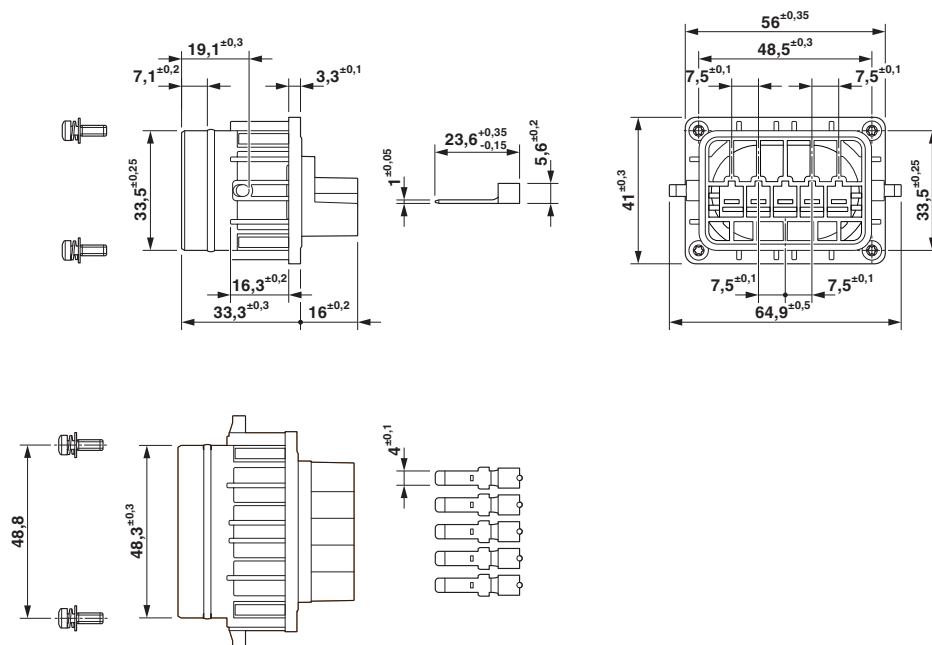
Disegno quotato
