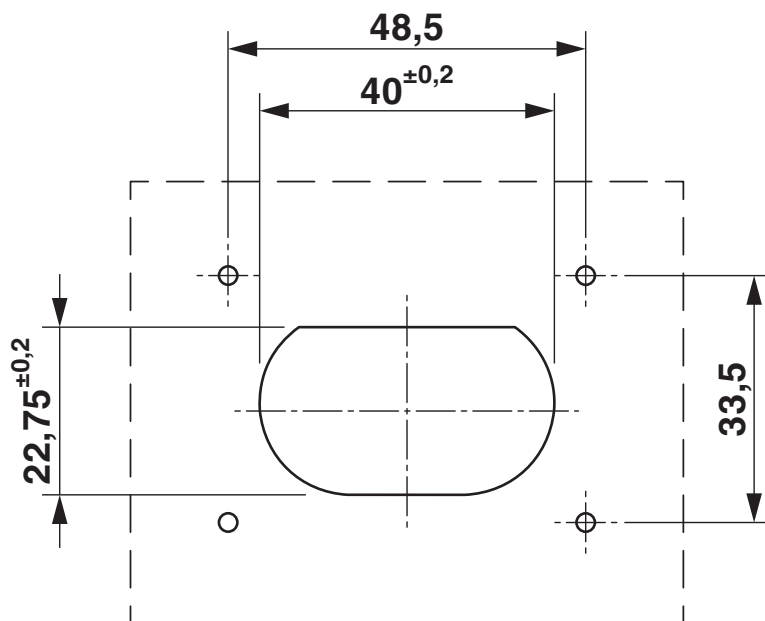
Dima di forat./geometria di pad di saldat.
