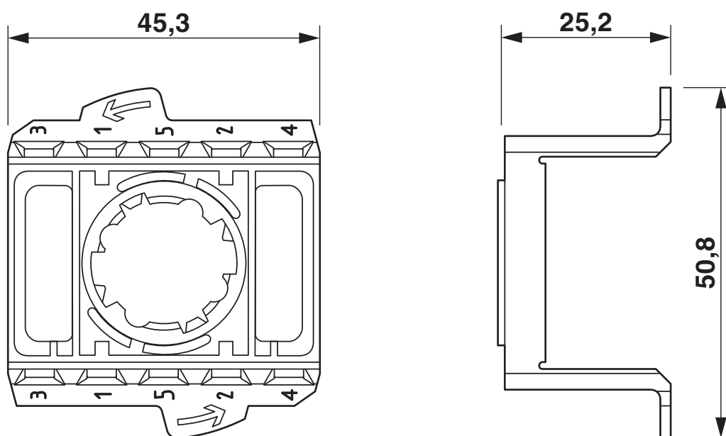
Disegno quotato
