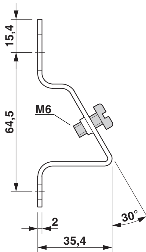
Disegno quotato
