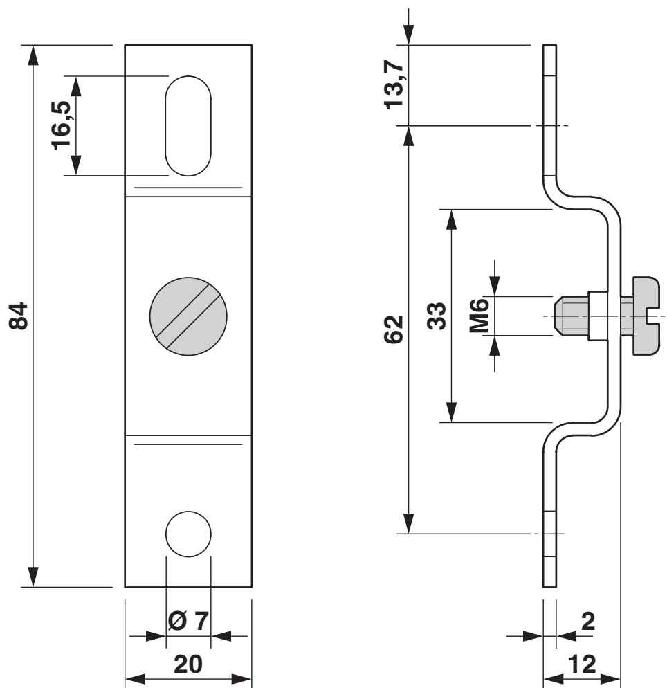
Disegno quotato
