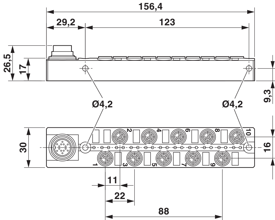
Disegno quotato
