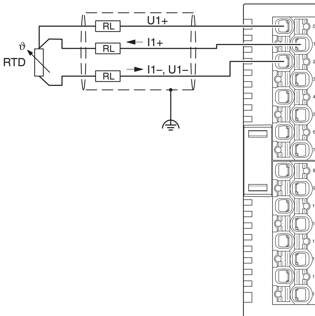
Disegno collegamento
