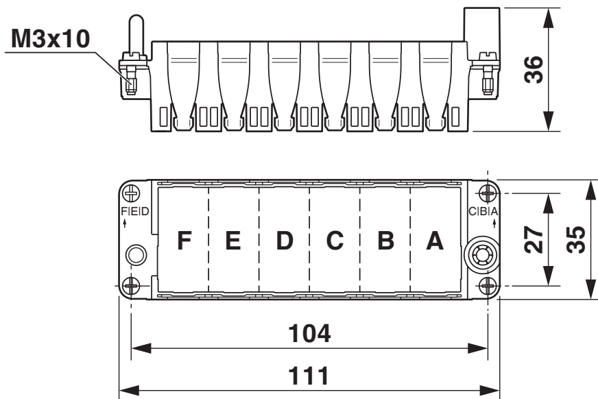
Disegno quotato
