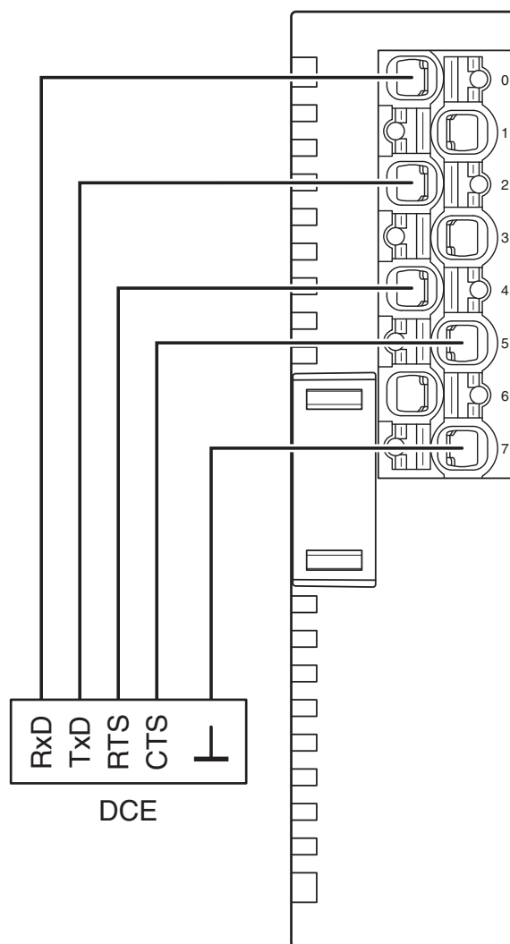
Disegno collegamento
