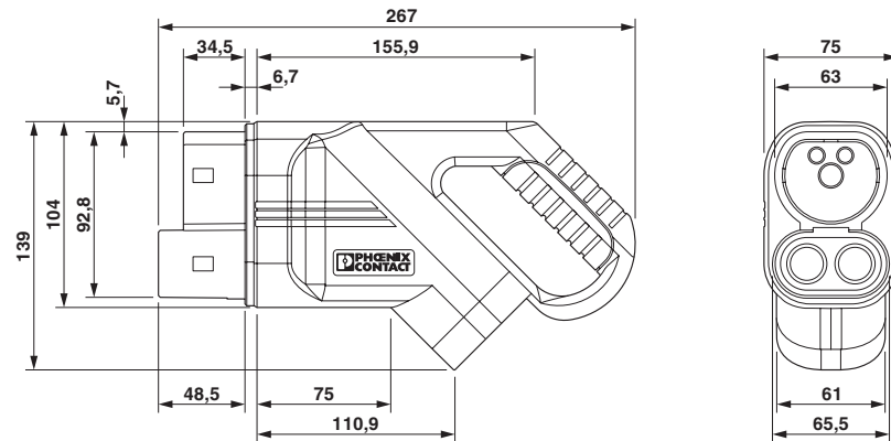
Disegno quotato
