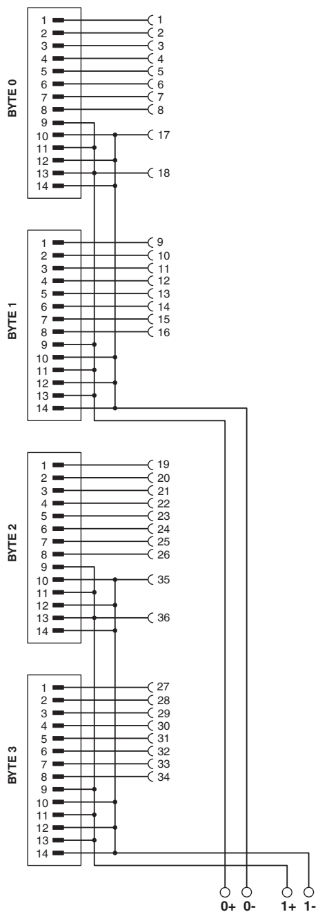
Schema di collegamento
