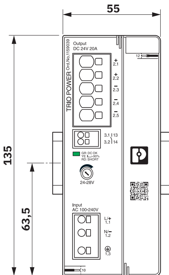
Disegno quotato
