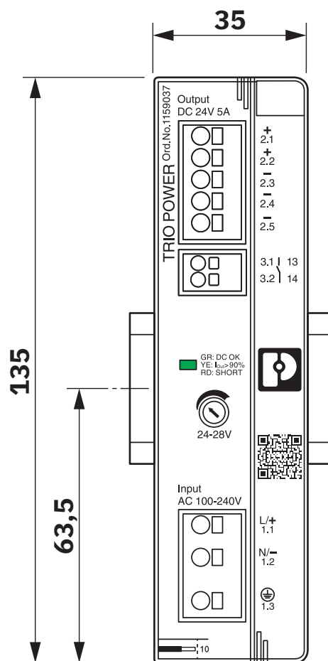
Disegno quotato
