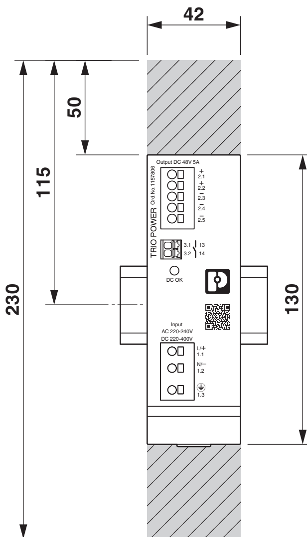
Disegno quotato
