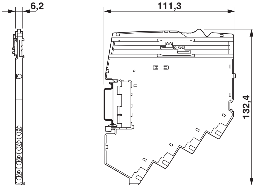
Disegno quotato
