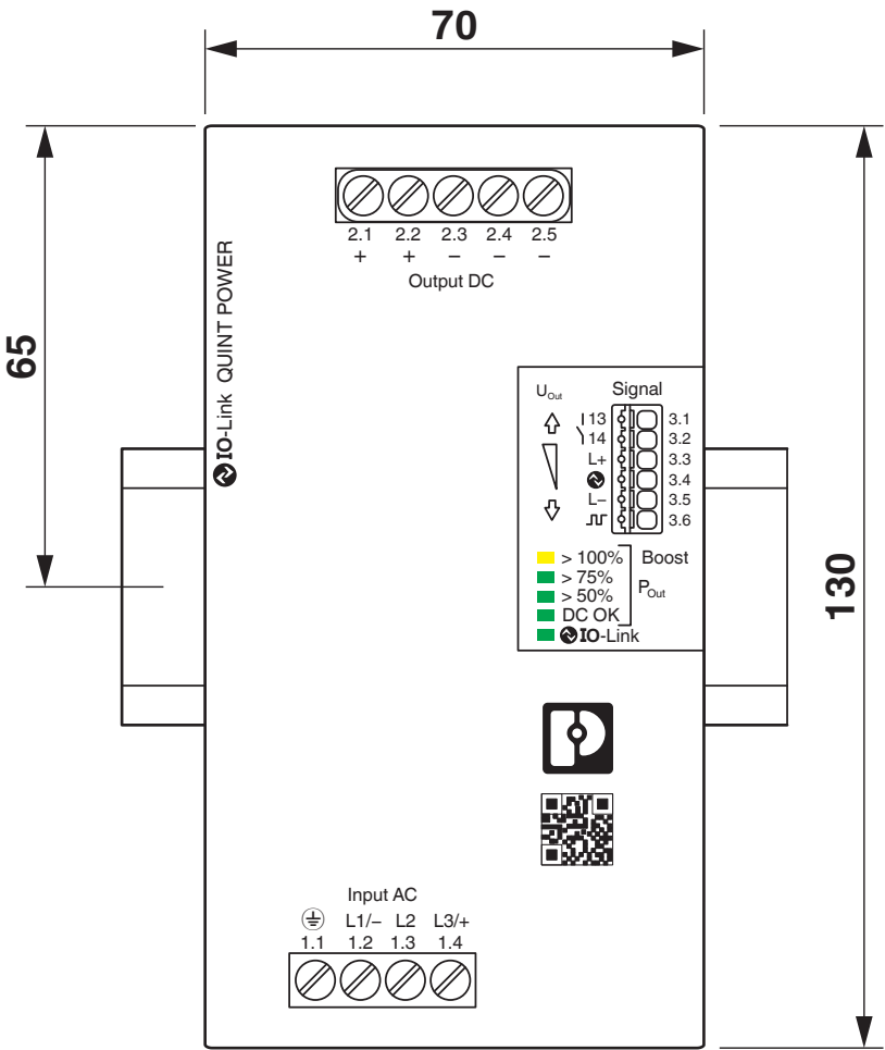
Disegno quotato
