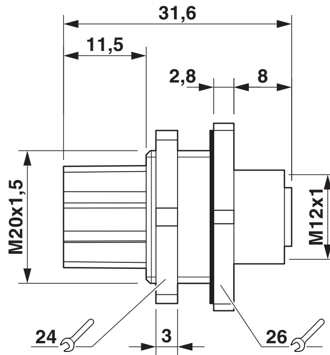
Disegno quotato
