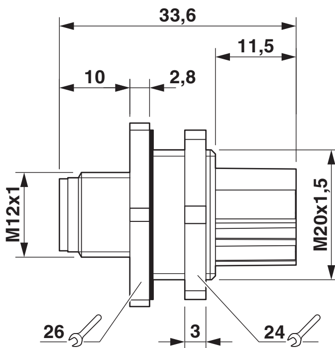
Disegno quotato
