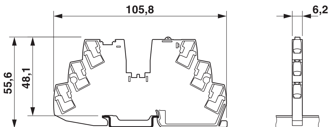
Disegno quotato
