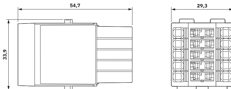
Disegno quotato
