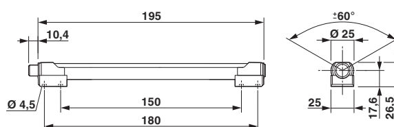
Disegno quotato
