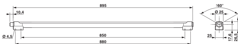
Disegno quotato
