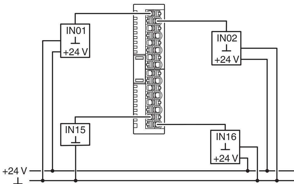
Disegno collegamento
