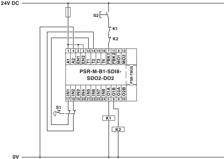
Disegno applicazione
