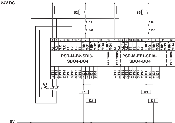
Disegno applicazione
