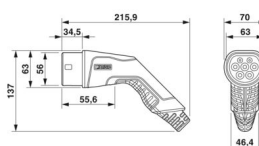
Connettore di ricarica del veicolo
