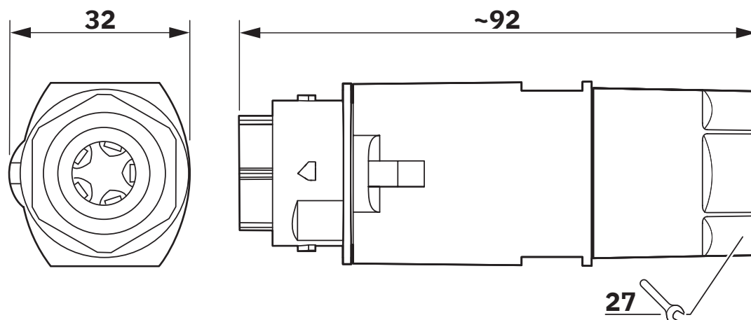
Disegno quotato
