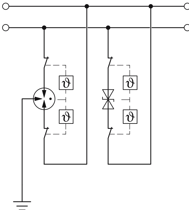
Disegno collegamento
