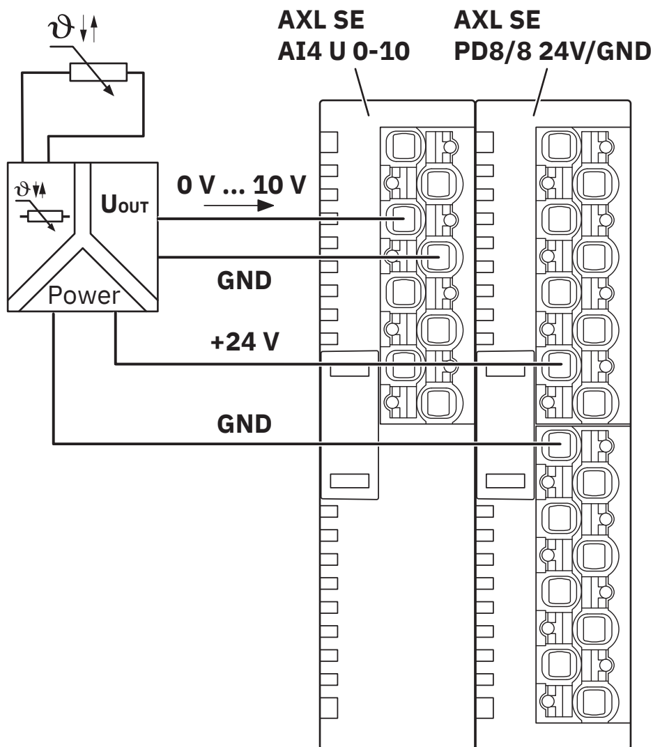
Disegno collegamento
