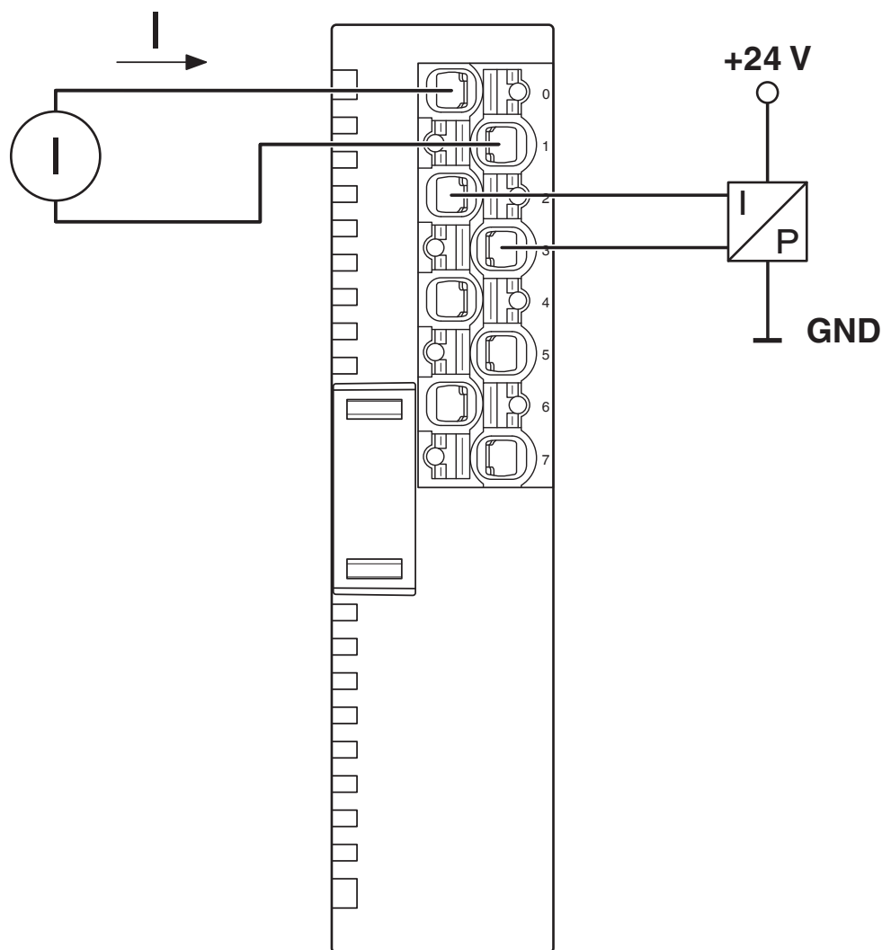
Disegno collegamento
