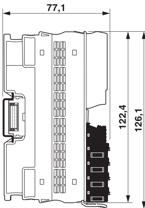
Disegno quotato
