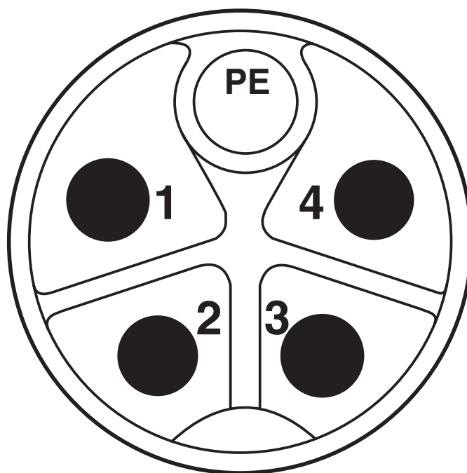
Pinning connettore M12, 4 poli+PE, codifica B, lato maschio
