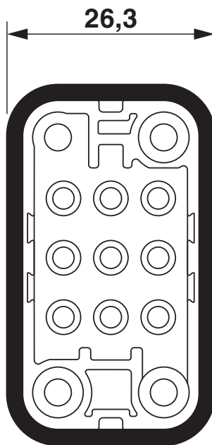
Disegno quotato HC-COM-8-EBUC
