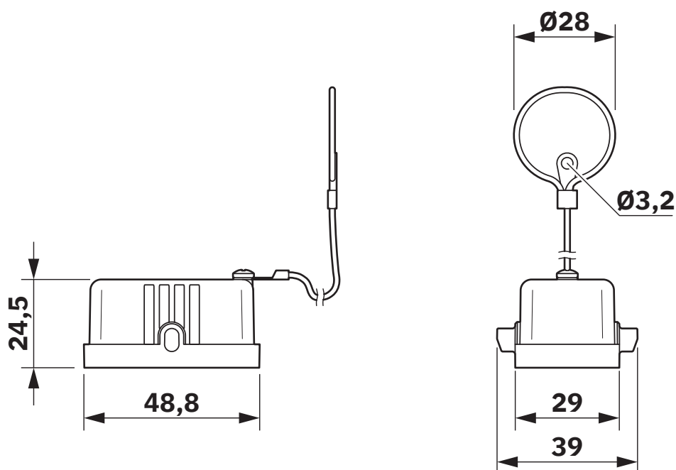
Disegno quotato
