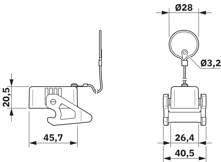
Disegno quotato
