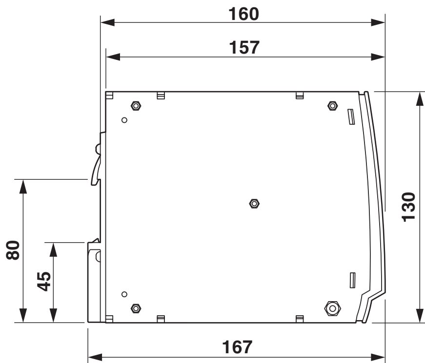
Disegno quotato
