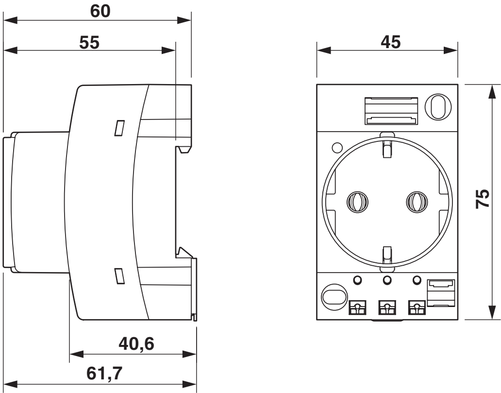
Disegno quotato
