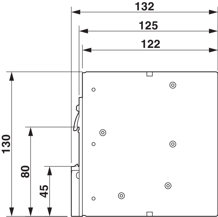
Disegno quotato
