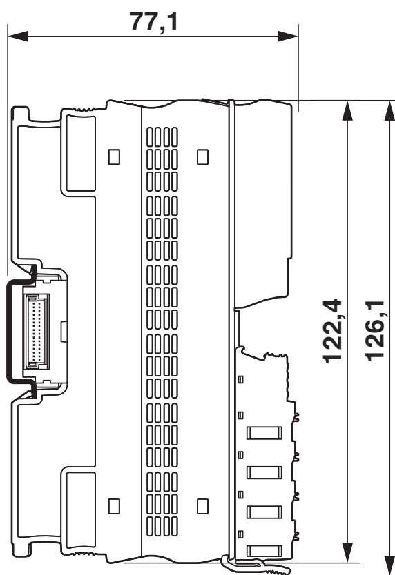
Disegno quotato
