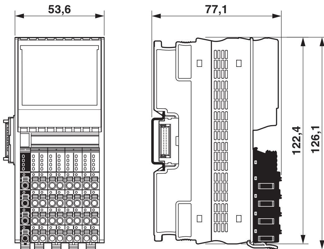
Disegno quotato
