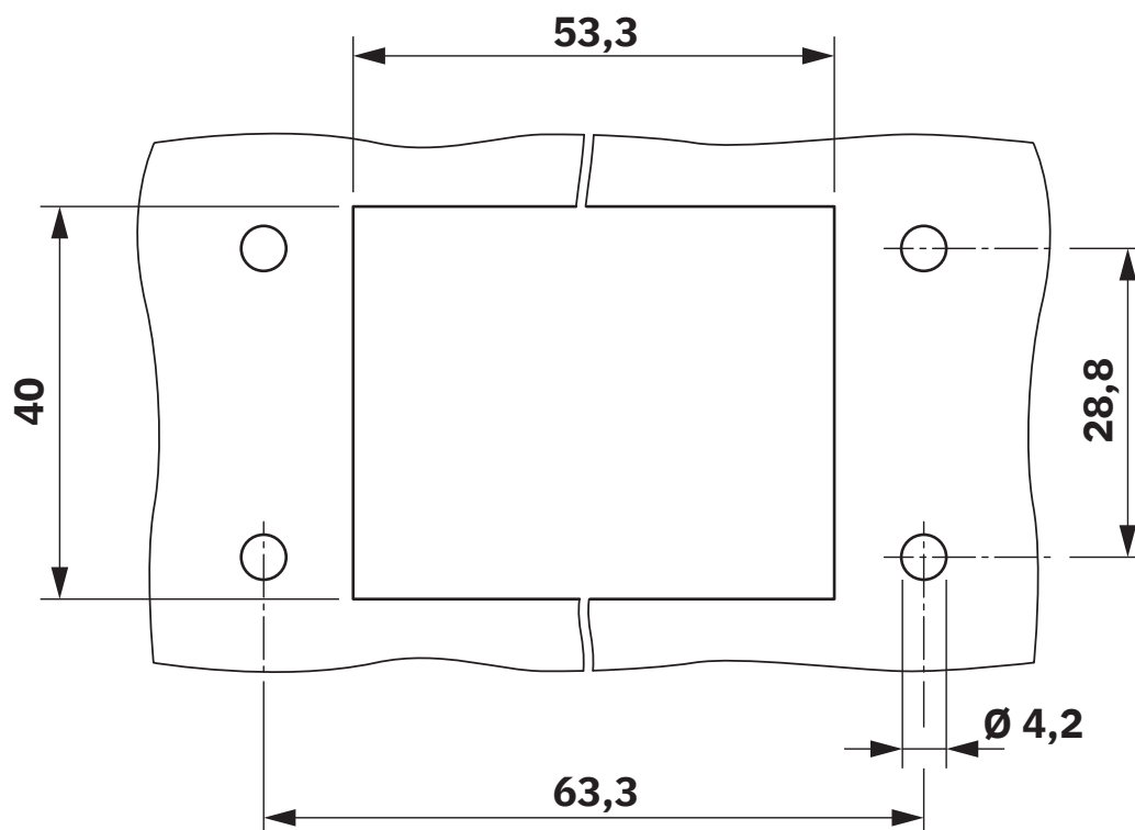
Disegno quotato
