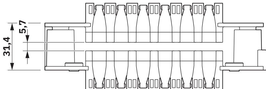
Disegno schematico Dockingframe
