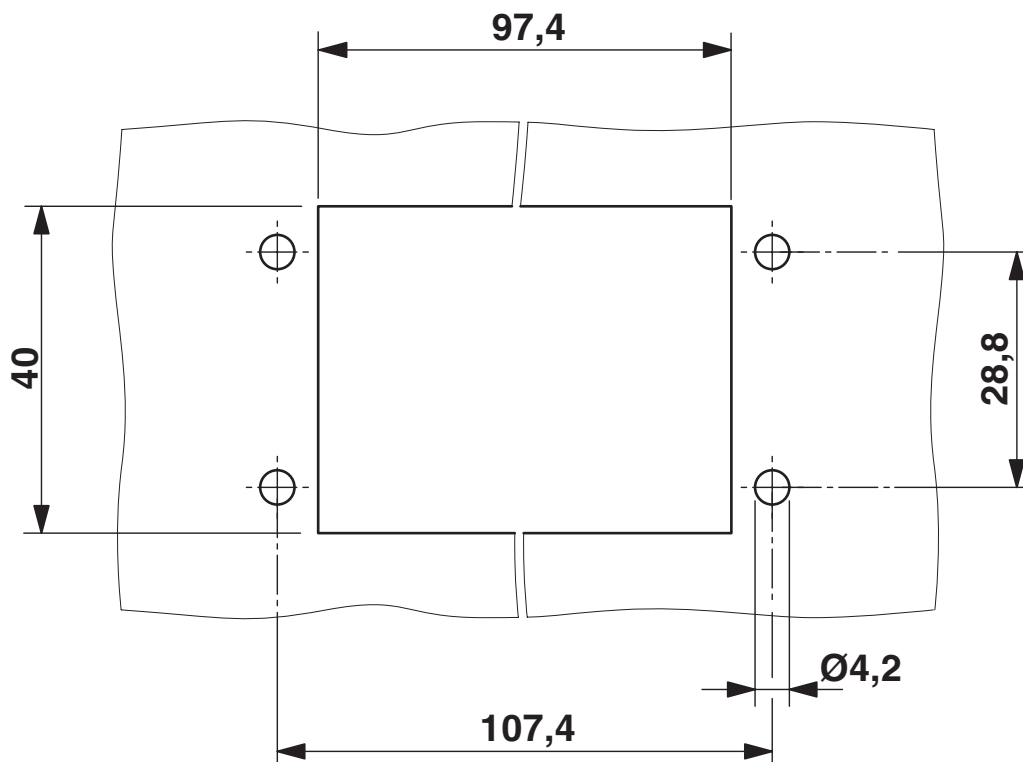
Disegno quotato
