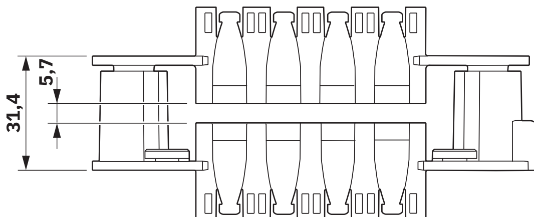
Disegno schematico Dockingframe
