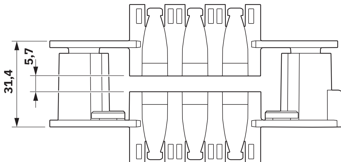
Disegno schematico Dockingframe
