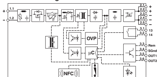
Diagramma a blocchi
